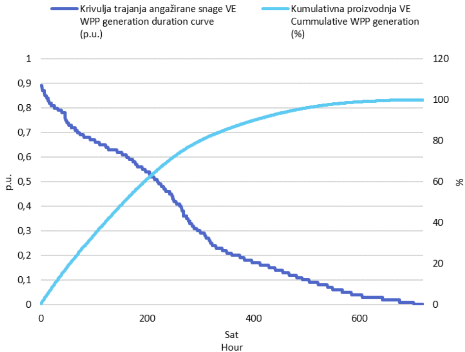
Slika 3 Krivulja trajanja angažirane snage svih VE i kumulativna proizvodnja VE u travnju 2022. godine u jediničnim vrijednostima
