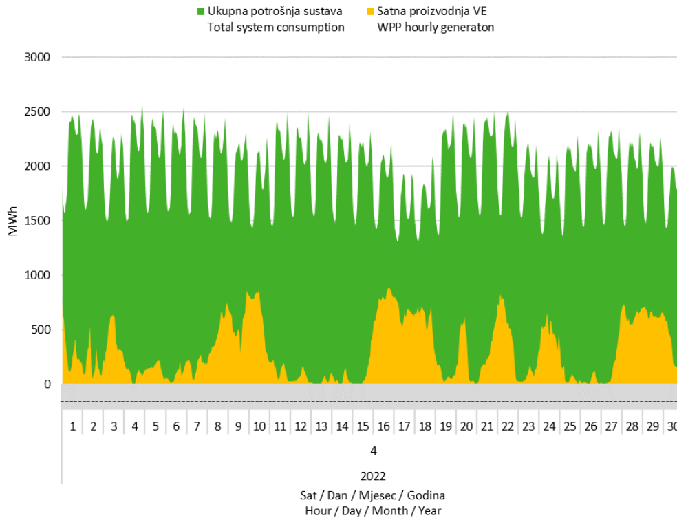
Slika 7 Usporedba satnog dijagrama opterećenja sustava i proizvodnje vjetroelektrana u travnju 2022. godine
