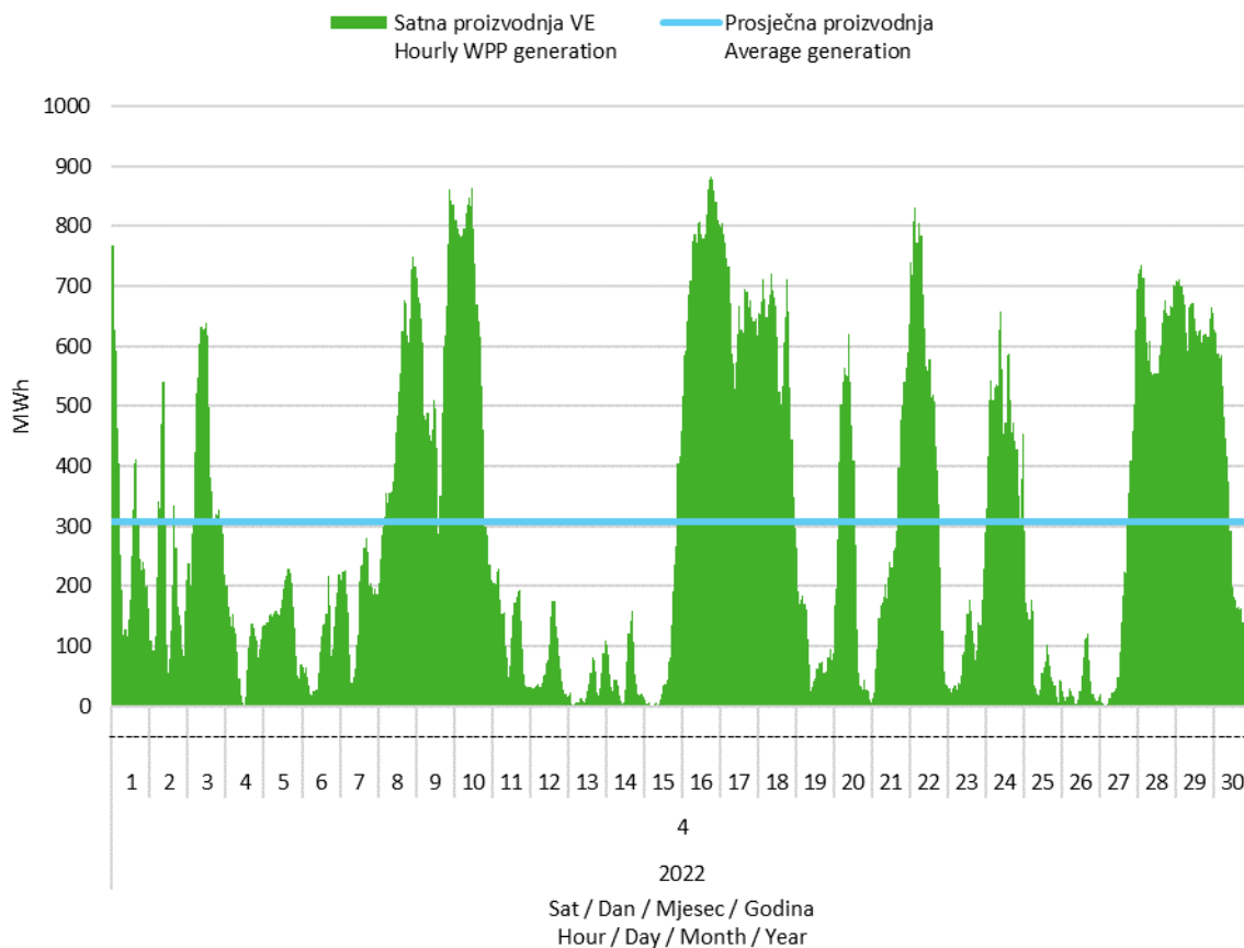
Slika 2 Satna proizvodnja svih vjetroelektrana u travnju 2022. godine
