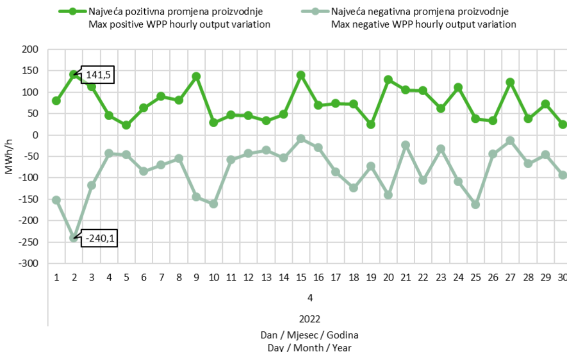
Slika 9 Maksimalna pozitivna i maksimalna negativna promjena satne proizvodnje VE u travnju 2022. godine
