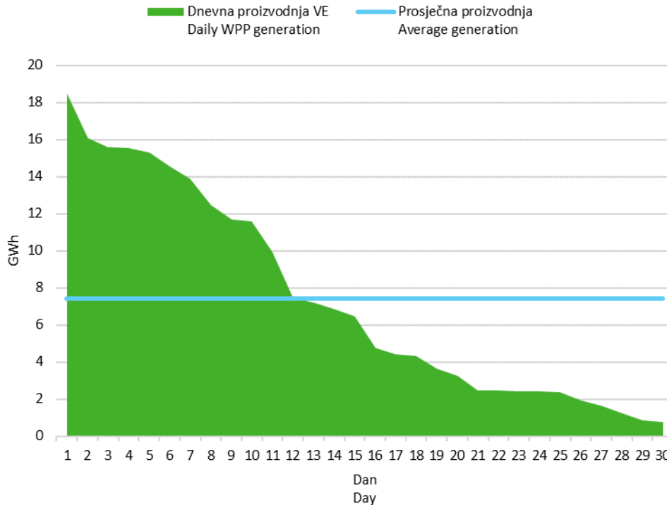
Slika 6 Krivulja trajanja dnevne proizvodnje vjetroelektrana u travnju 2022. godine
