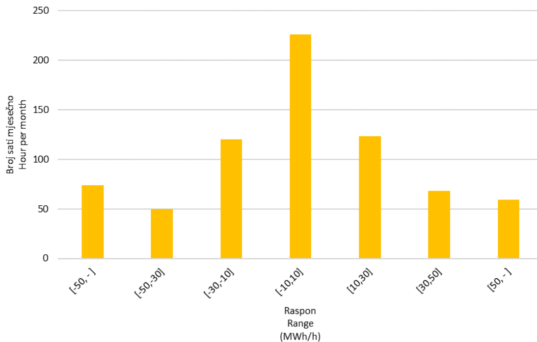
Slika 10 Statistička raspodjela satnih promjena proizvodnje VE u travnju 2022. godine
