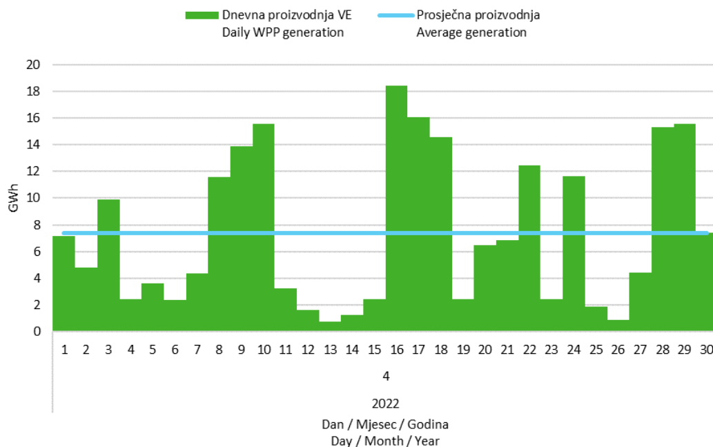
Slika 5 Dnevna proizvodnja svih vjetroelektrana u travnju 2022. godine
